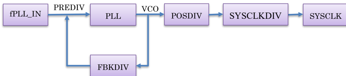
图 4-2 系统时钟示意图
