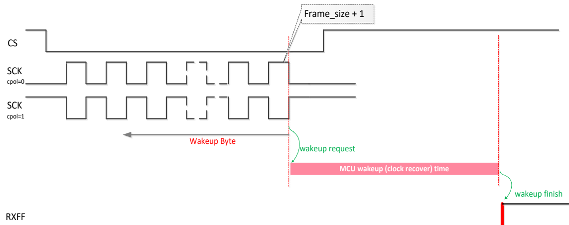
图 18-10 唤醒序列
