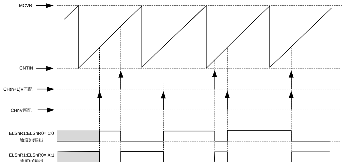
图 11-24 CH(n+1)V 在下一周期匹配的输出波形
