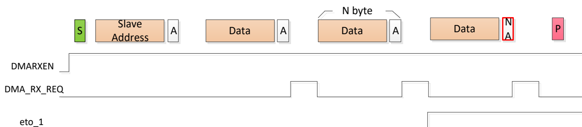
图 17-12 从机接收器
