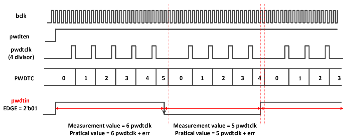
图 12-7 PWDTC 计数器和计数错误
