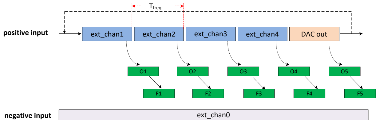
图 10-2 轮询模式工作流程图
