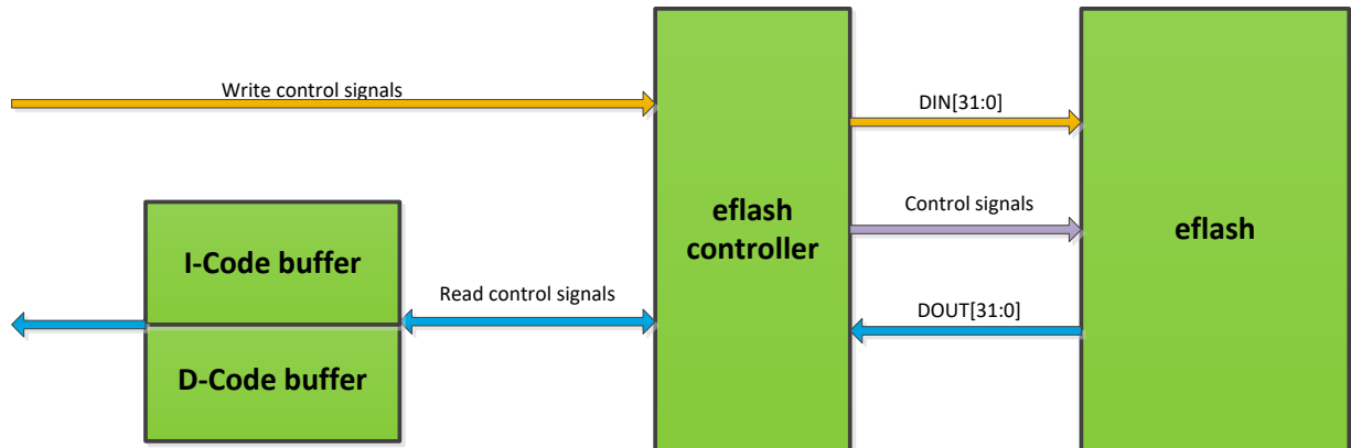
图 22-2 eflash 和 eflash 控制器数据流
