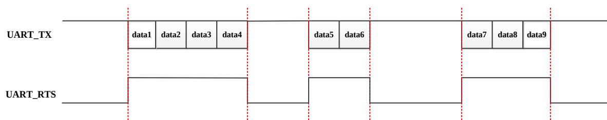
图 8-8 多字节数据传输
