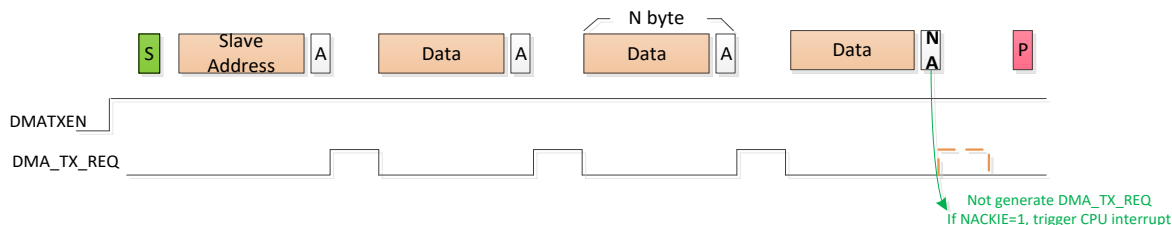
图 17-11 从机发送器
