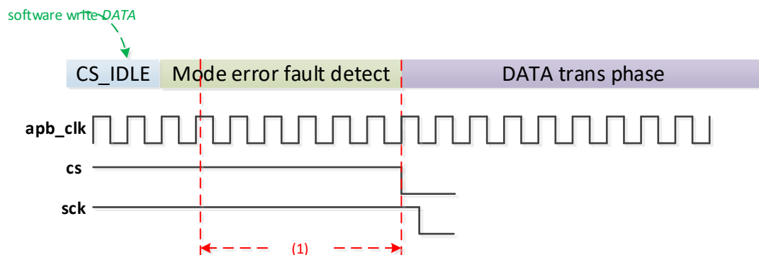
图 18-9 模式故障检测限制
