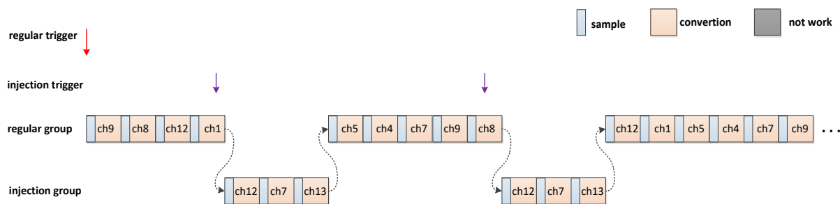
图 9-13 Mode 5 注入组扫描模式工作流程
