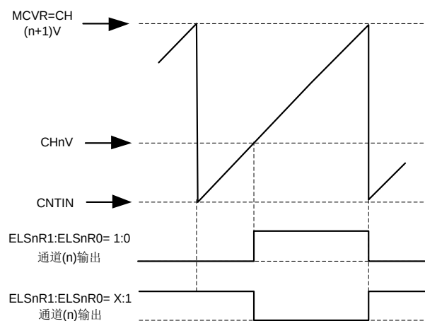
图 11-12 (CNTIN &lt; CHnV &lt; MCVR) &amp; (CH(n+1)V = MCVR)条件下输出波形
