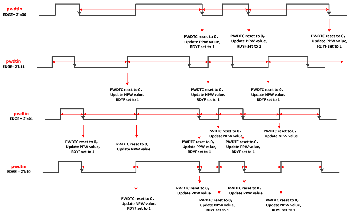
图 12-2 四种基本测量模式(HALLEN=0)
