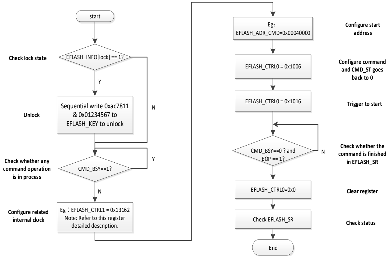
图 22-8 选项字节擦除命令操作流程
