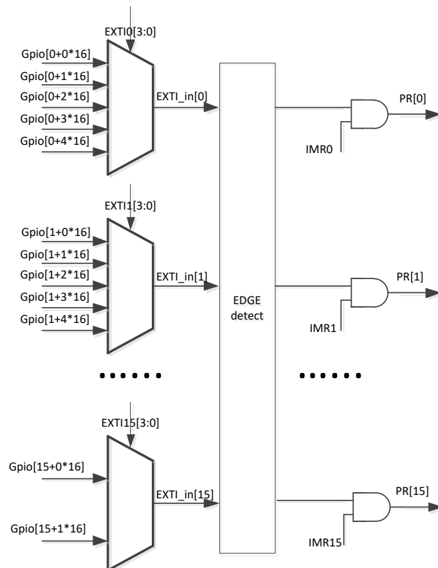
图 16-2 GPIO 外部中断
