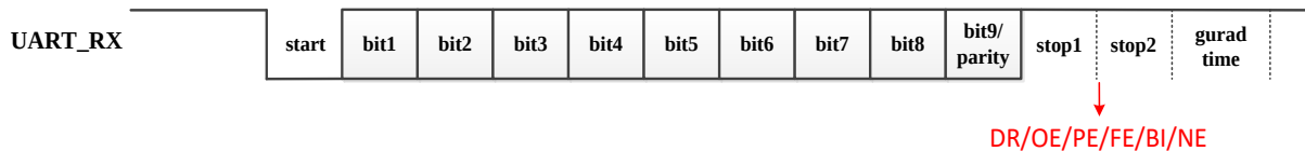
图 8-3 UART 接收器流程
