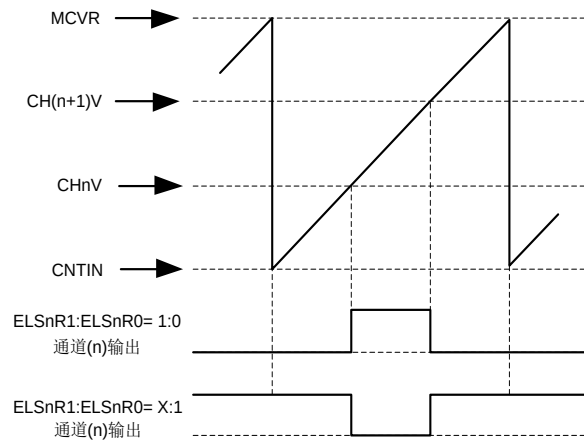
图 11-11 (CNTIN &lt; CHnV/CH(n+1)V &lt; MCVR) &amp; (CHnV &lt; CH(n+1)V)条件下输出波形
