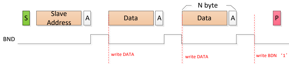
图 17-13 主机写从机模式的 BND 序列
