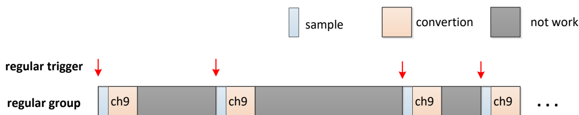
图 9-7 Mode 1 工作流程
