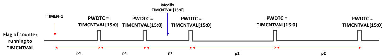
图 12-9 TIMEN=1 期间修改 TIMLDVAL
