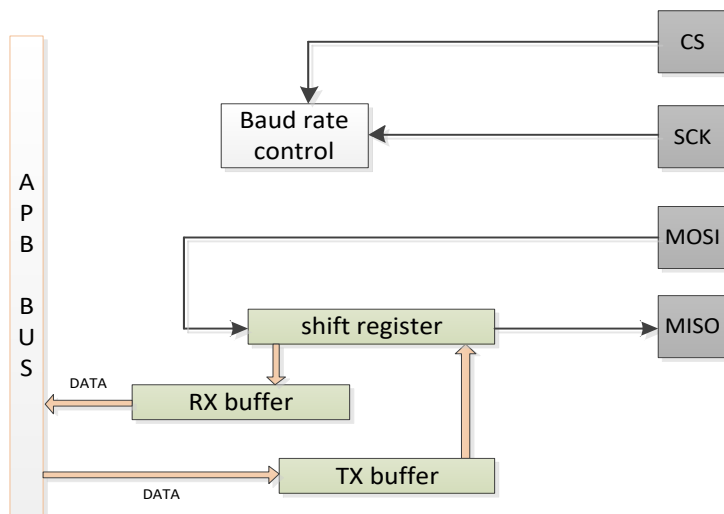
图 18-4 从机数据流
