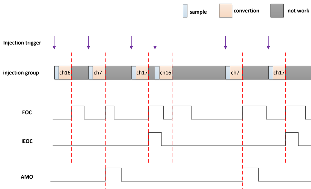
图 9-23 情形 3 下的三个标志行为
