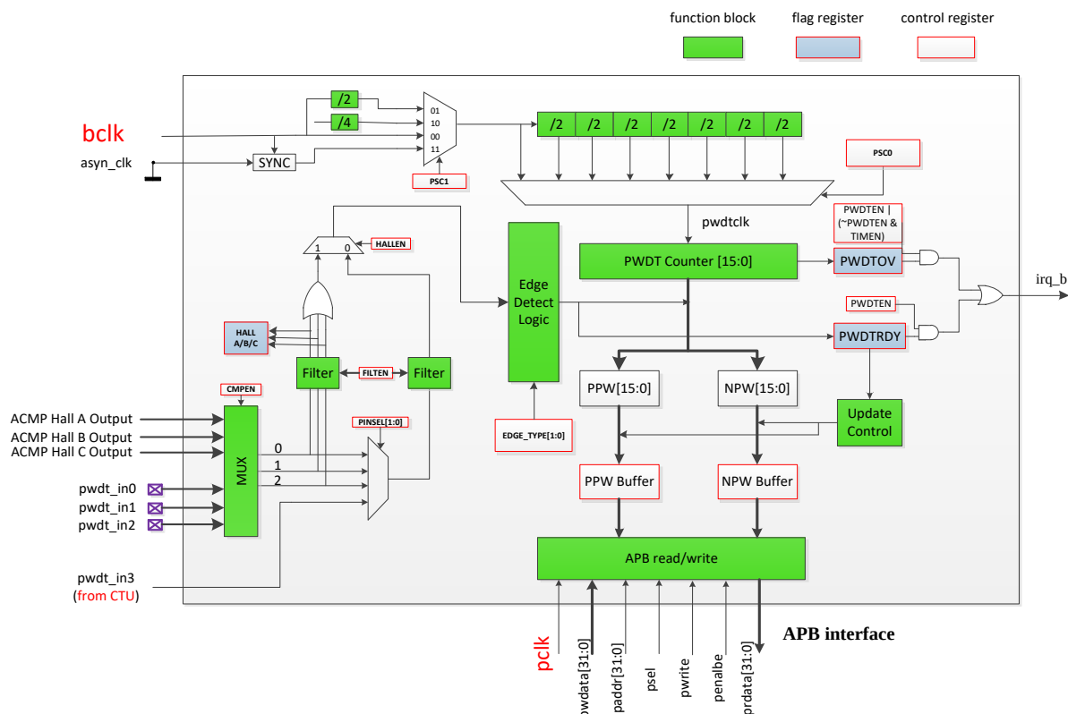
图 12-1 PWDT 结构框图
