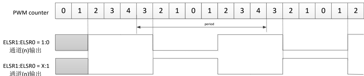
图 11-19 CHn 匹配点 DIR=1(Up)，CH(n+1)匹配点 DIR=0(Down)
