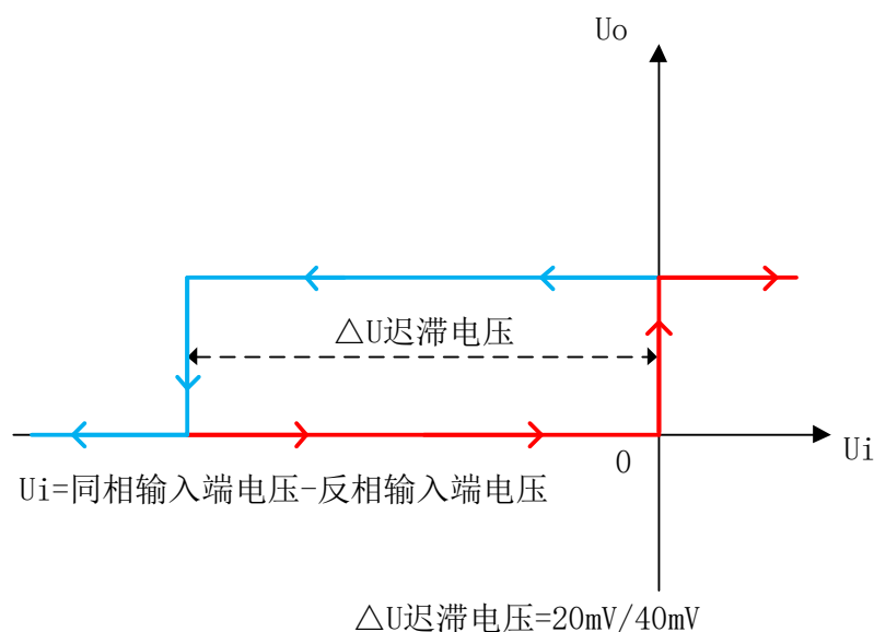
图 10-3 迟滞工作原理
