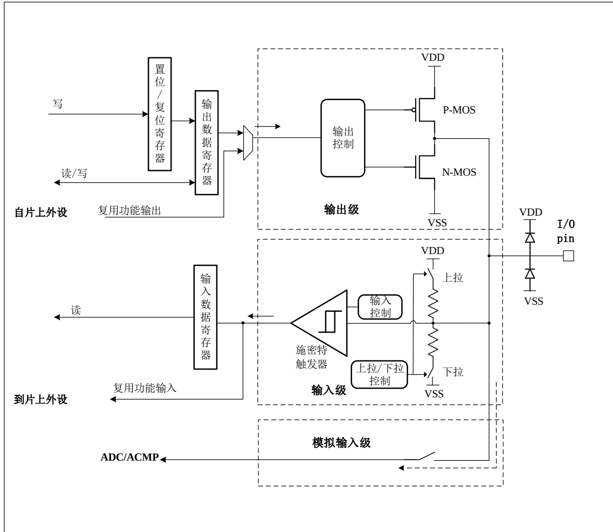
图 16-1 GPIO 结构框图
