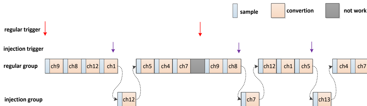
图 9-11 Mode 3 注入组间隔模式工作流程
