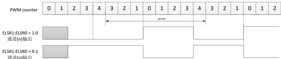
图 11-20 CHn 匹配点 DIR=0(Down)，CH(n+1)匹配点 DIR=1(Up)
