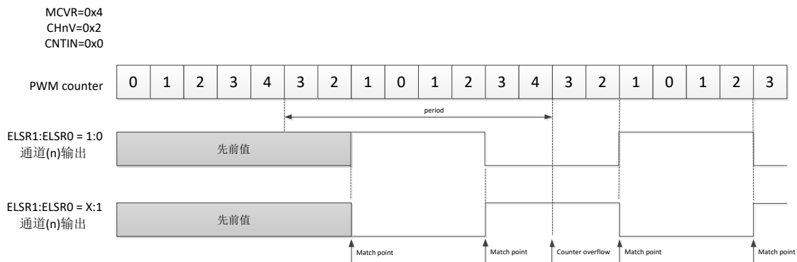
图 11-9 CPWM 波形
