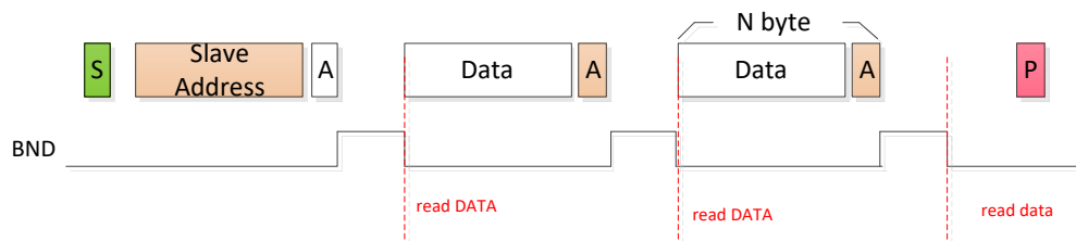
图 17-14 主机读从机模式的 BND 序列
