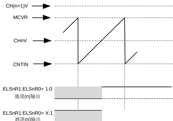
图 11-16 (CH(n+1)V > MCVR)且(CNTIN < CHnV < MCVR)条件下输出波形
