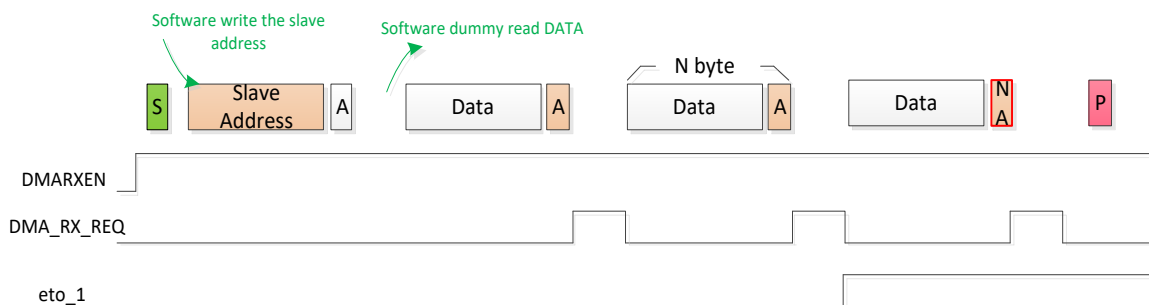
图 17-10 主机接收器
