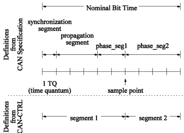
图 7-5 CAN 位定时
