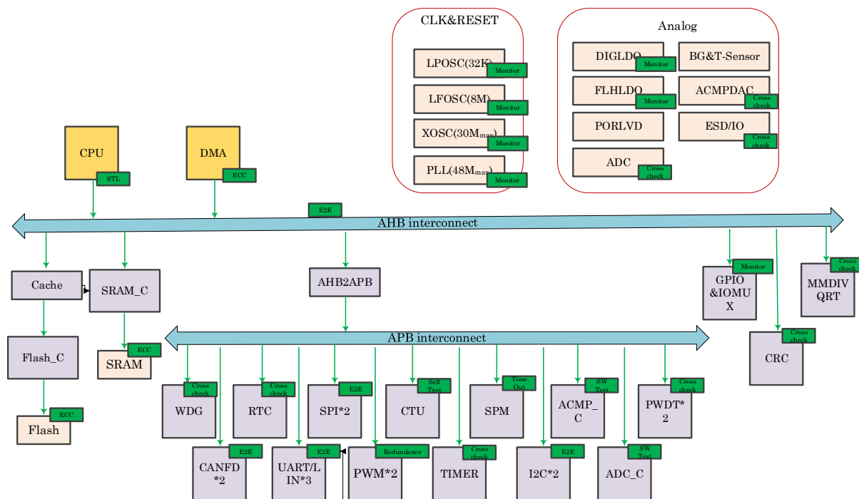
图 26-1 功能安全结构图
