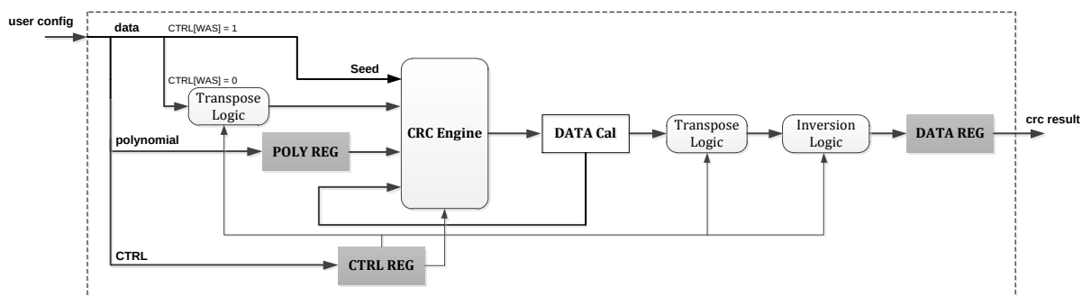
图 15-1 CRC 结构框图
