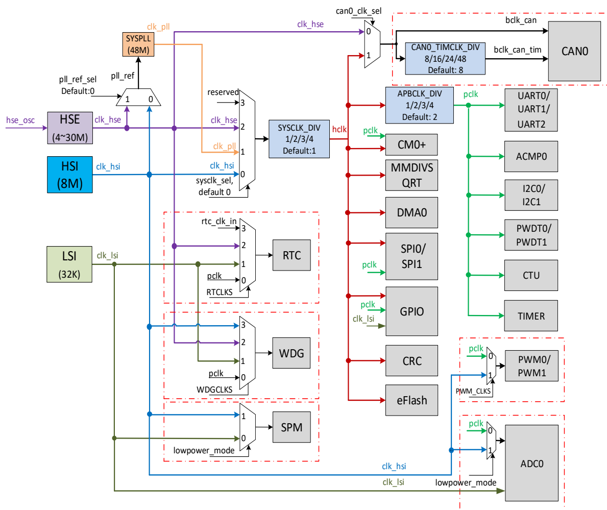
图 4-1 时钟控制结构
