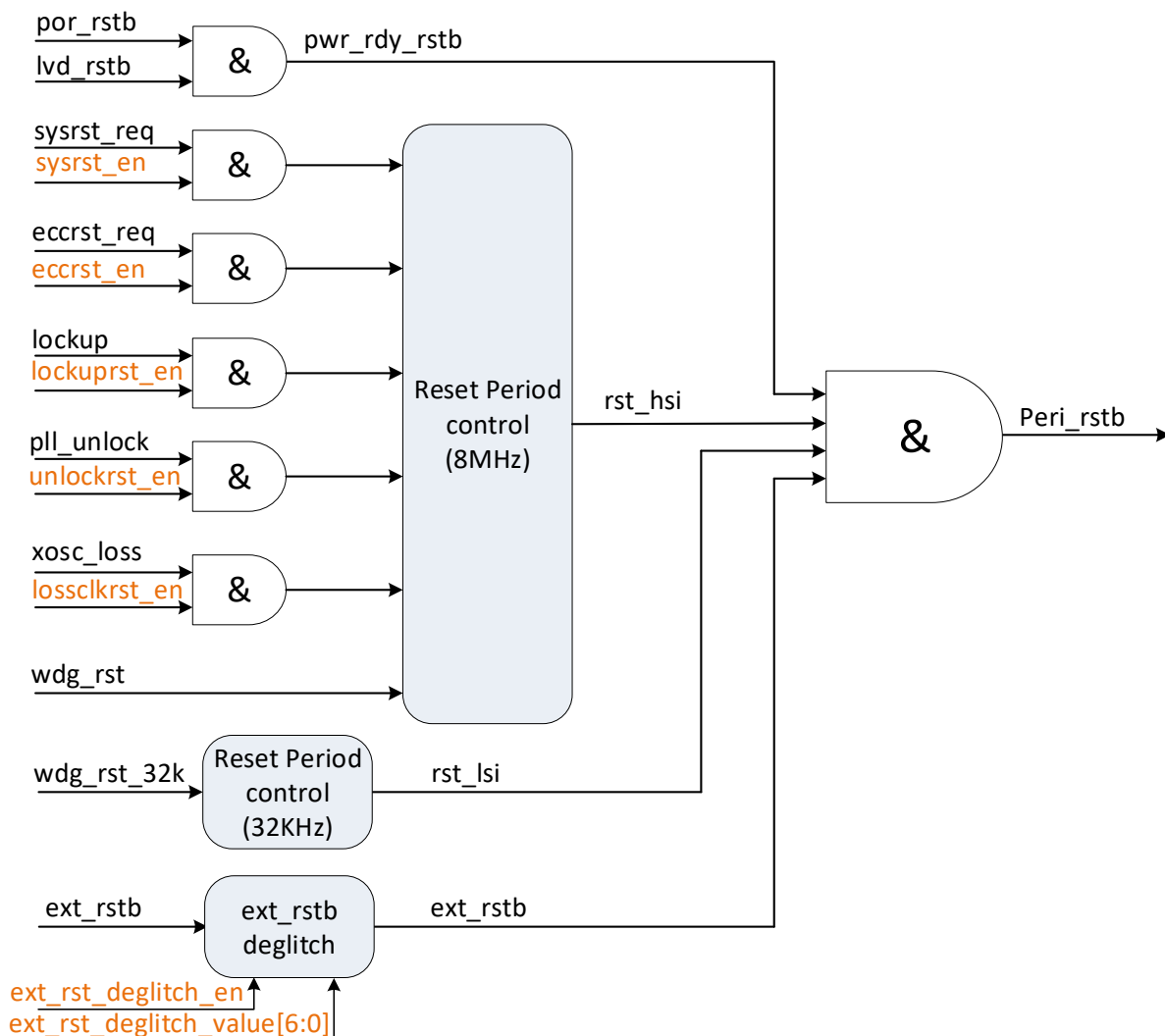
图 3-1 Reset 模块结构框图
