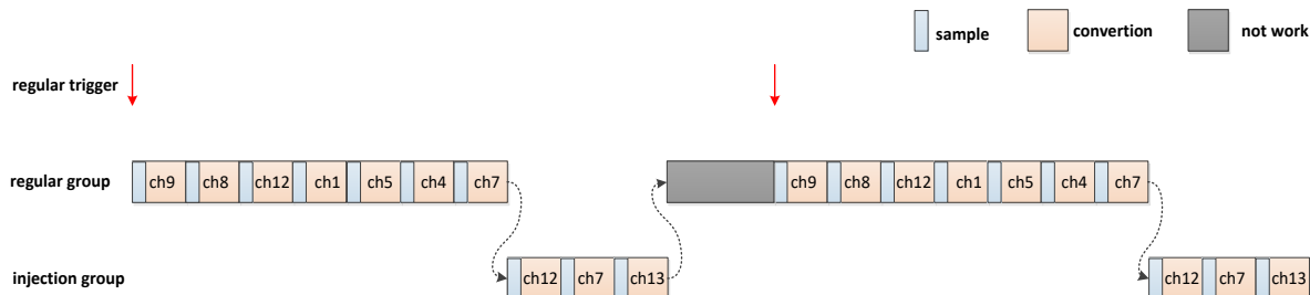
图 9-12 Mode 4 工作流程
