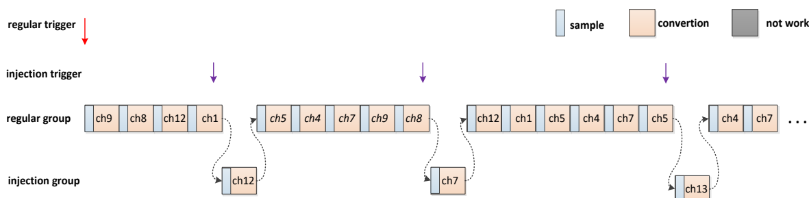
图 9-15 Mode 5 注入组间隔模式工作流程
